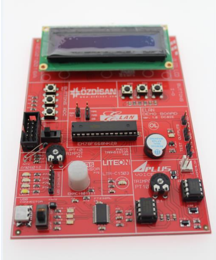
Şekil 2: Elan Demo Board
