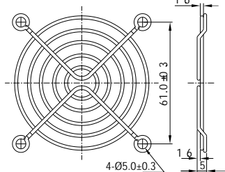
MG 07 For 70mm Fan
