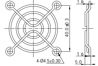
MG 05 For 50mm Fan
