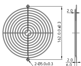
MG 15 For 150mm Fan
