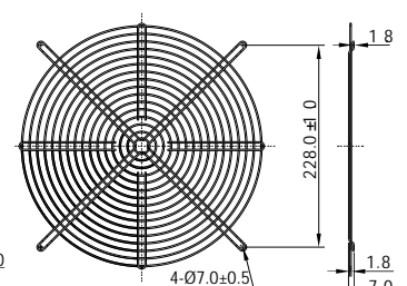
MG 25 For 250mm Fan
